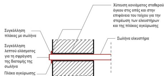
Σχέδιο 2: Σκαρίφημα που παρουσιάζει τον τρόπο τοποθέτησης των δεκάμετρων ελκυστήρων.
