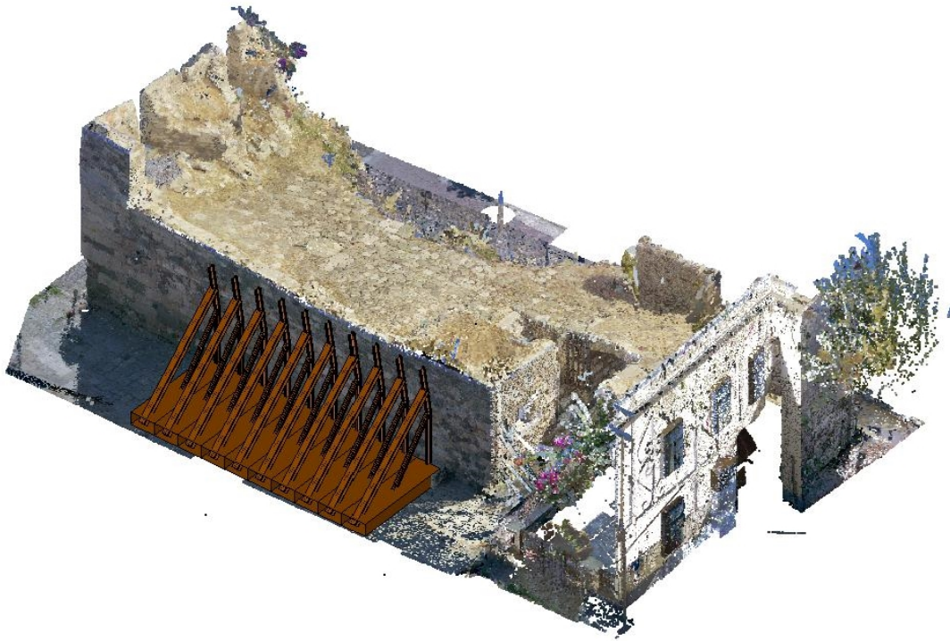
Σχέδιο 1: Τρισδιάστατη αποτύπωση του ΝΑ Προμαχώνα
