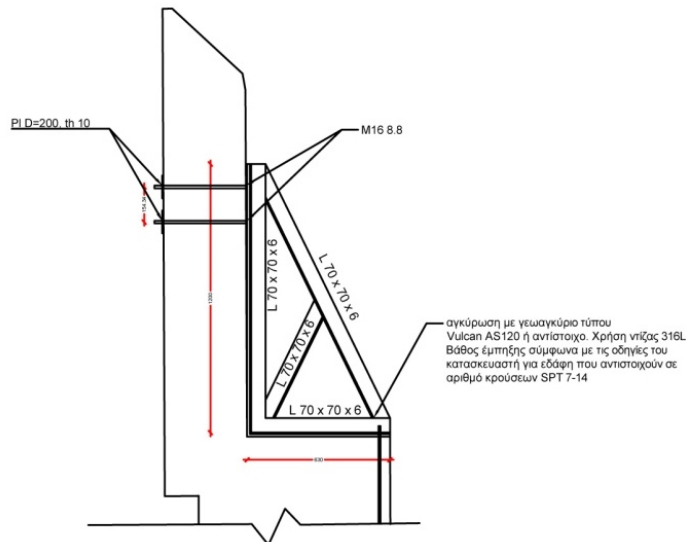
Σχέδιο 8: Σκαρίφημα τριγωνικής αντηρίδας Σκοπιάς.
