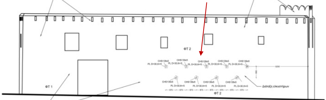
1 Όψη τοίχων ΦΤ1 και ΦΤ2 1 : 100
