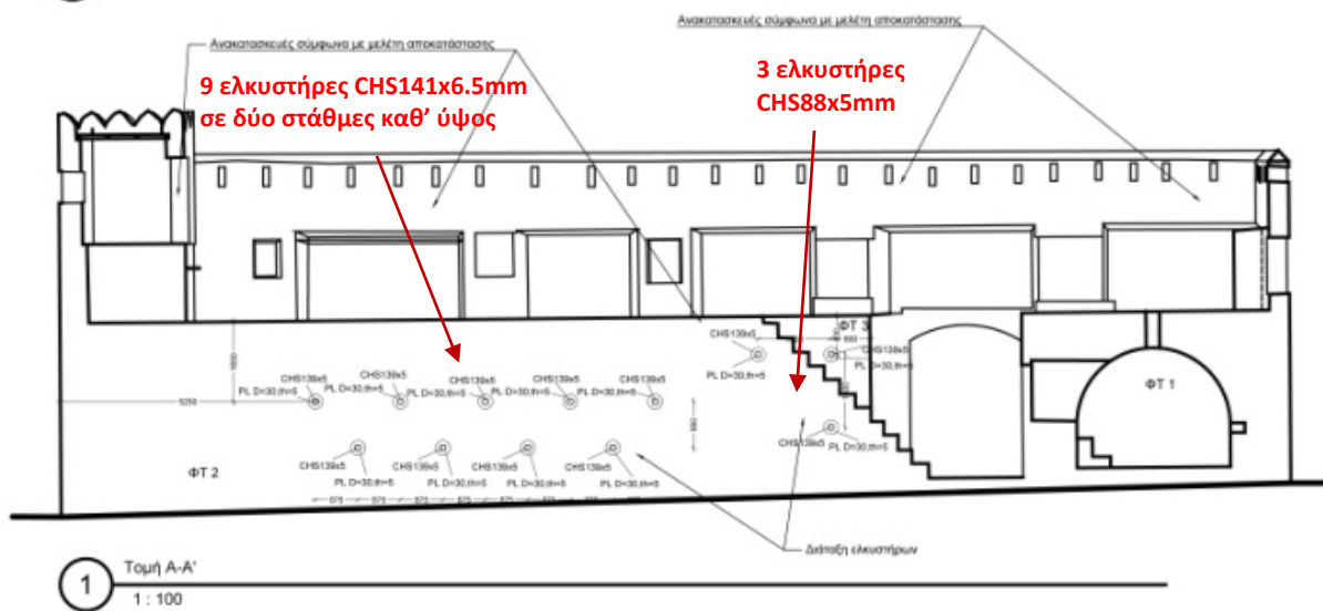
Σχέδιο 6: Τομές ΝΑ Προμαχώνα.
