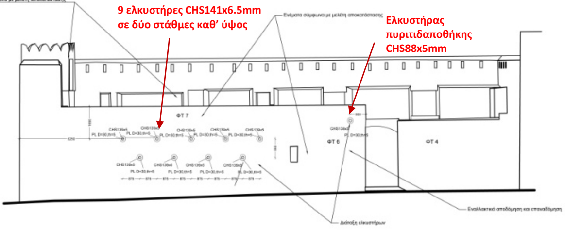
2 Όψη τοίχων ΦΤ6 και ΦΤ7 1 : 100
