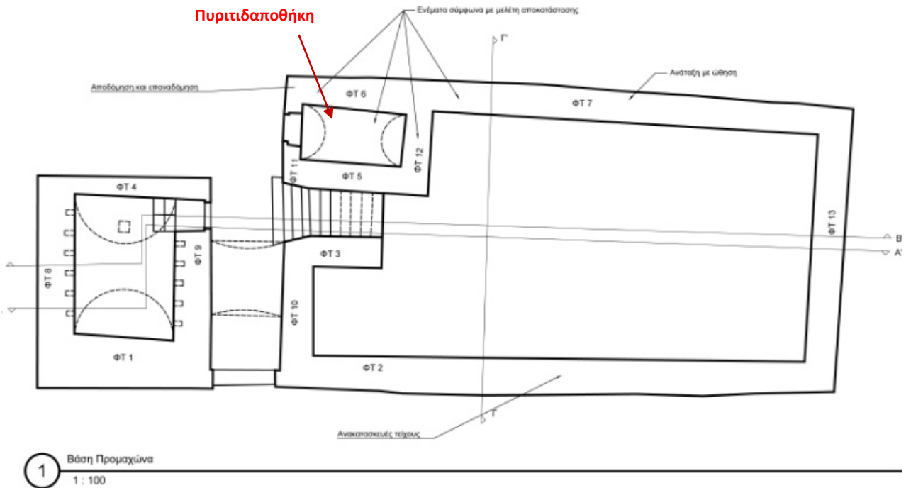
Σχέδιο 3: Κατόψεις ΝΑ Προμαχώνα σε δύο στάθμες
